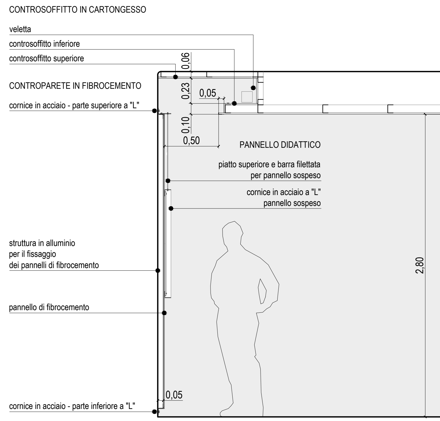
PARTI - SEZIONE TIPO
