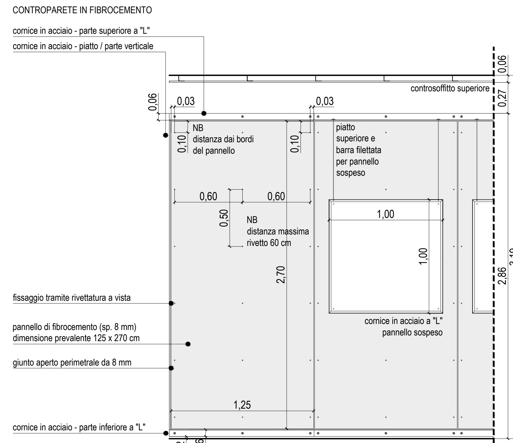
PARTI - PROSPETTO TIPO
