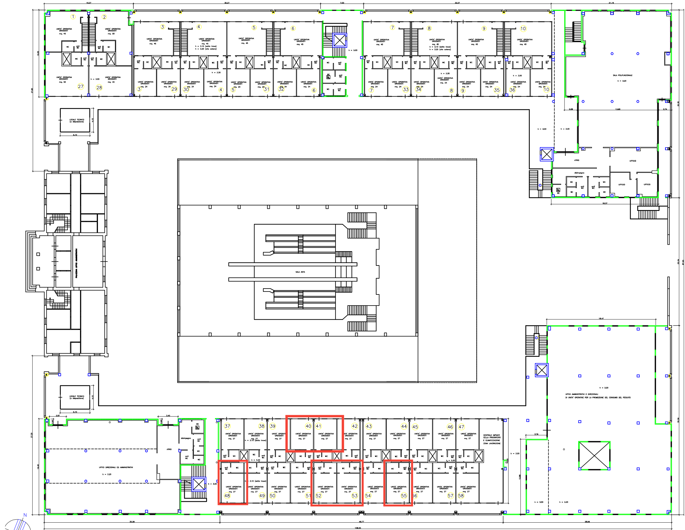
PIANTA PRIMO PIANO MERCATO ITTICO
